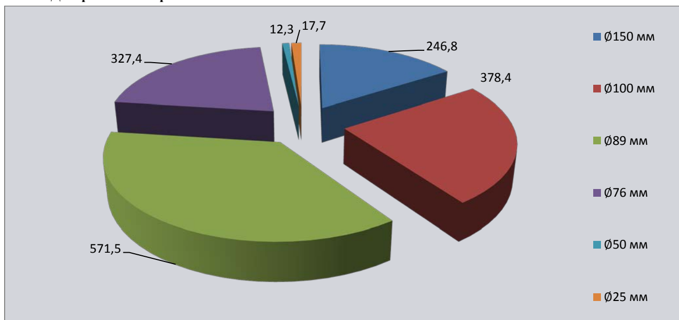
Диаграмма №1 Протяженность тепловых сетей котельной с.Чажемто
