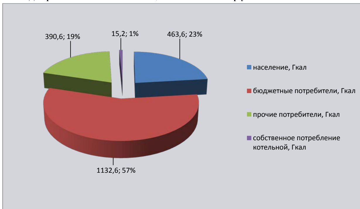
Диаграмма 2. Баланс тепловой мощности и тепловых нагрузок котельной с.Чажемто.
